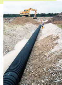
Drenažni sustav
